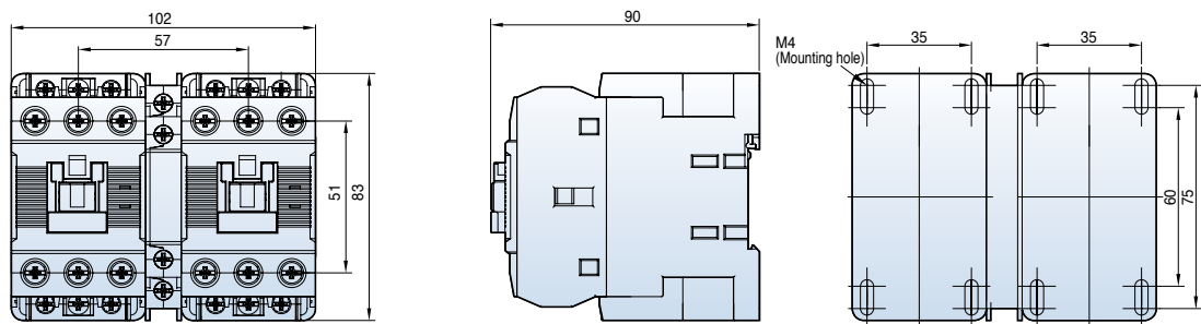
MC-32aR~40aR AC
