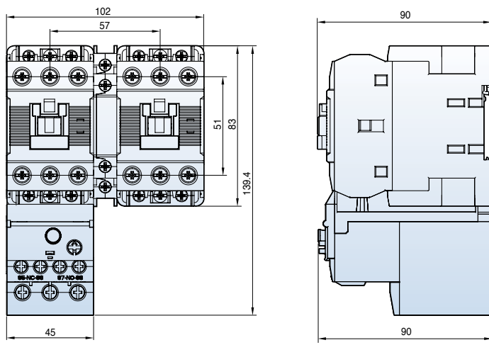
MS-32aR~40aR AC
