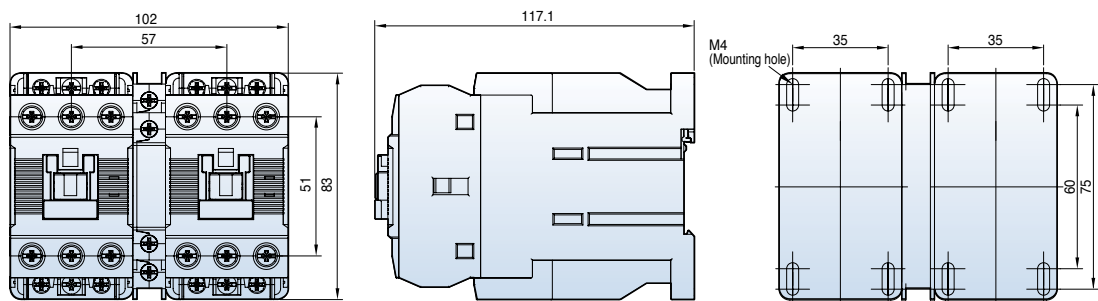
MC-32aR~40aR DC
